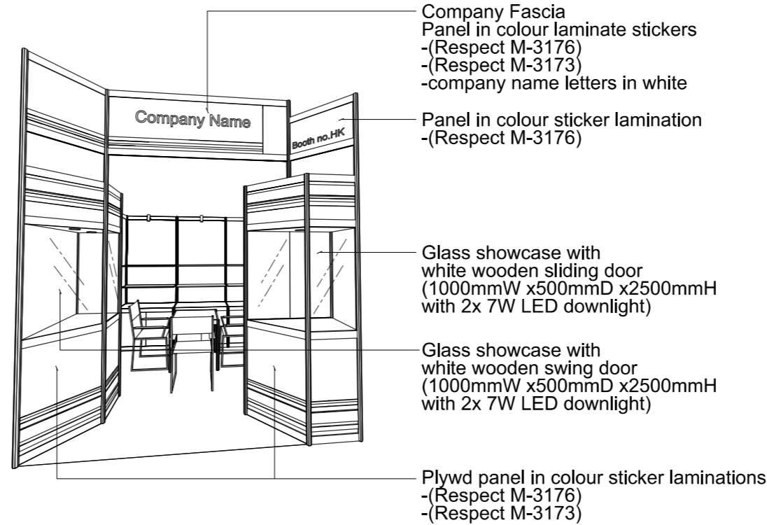
PERSPECTIVE N.T.S.
